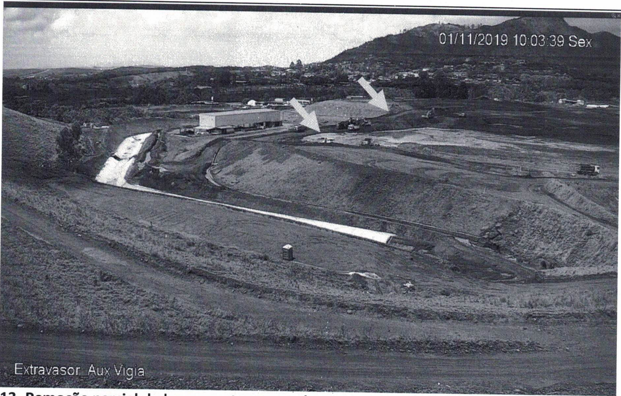
Foto 13- Remoção parcial do barramento e terraplanagem final de todo o reservatório extinguindo a capacidade de armazenamento de água e rejeito
