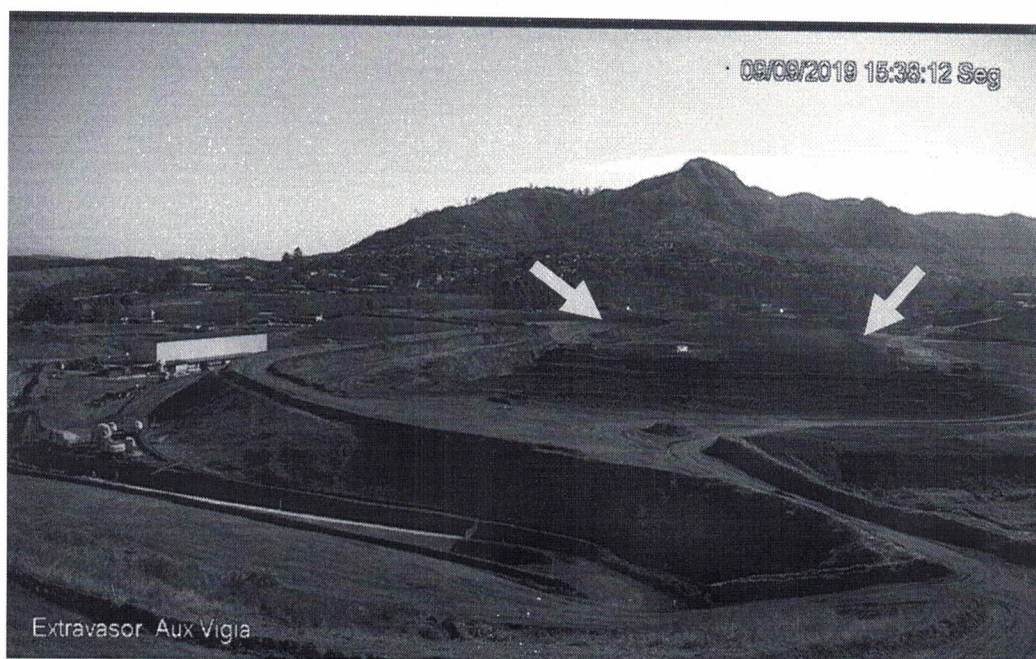
Foto 10- Vista superior do sequenciamento dos trabalhos de escavação e remoção parcial do rejeito a montante
