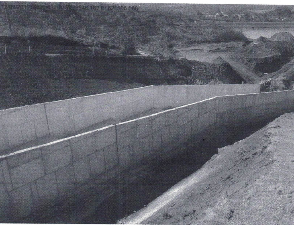
Foto 8- Trecho final do canal extravasor concretado
