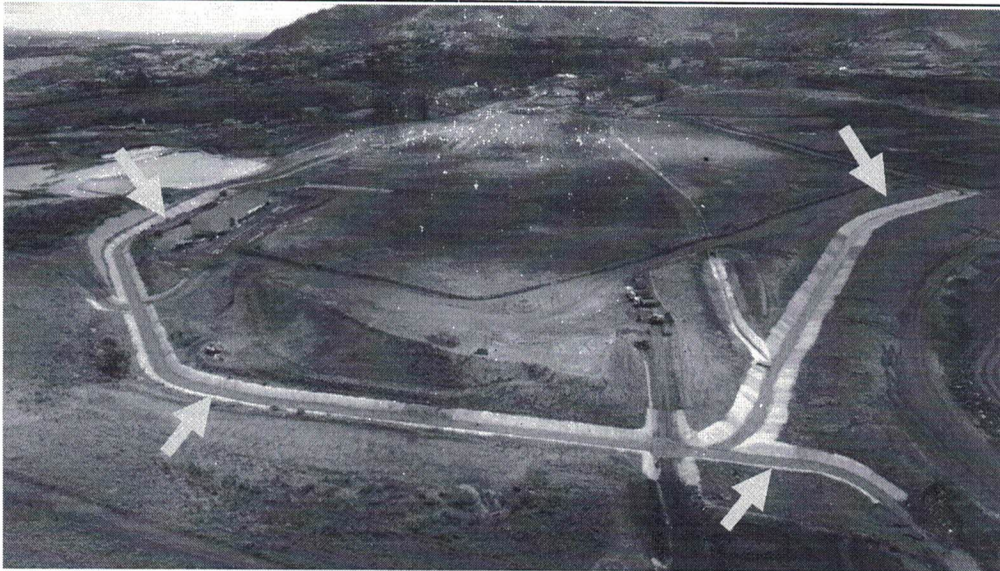
Foto 17- Vista superior do canal de cintura e novo vertedouro implantado para desvio das contribuições das drenagens adjacentes
