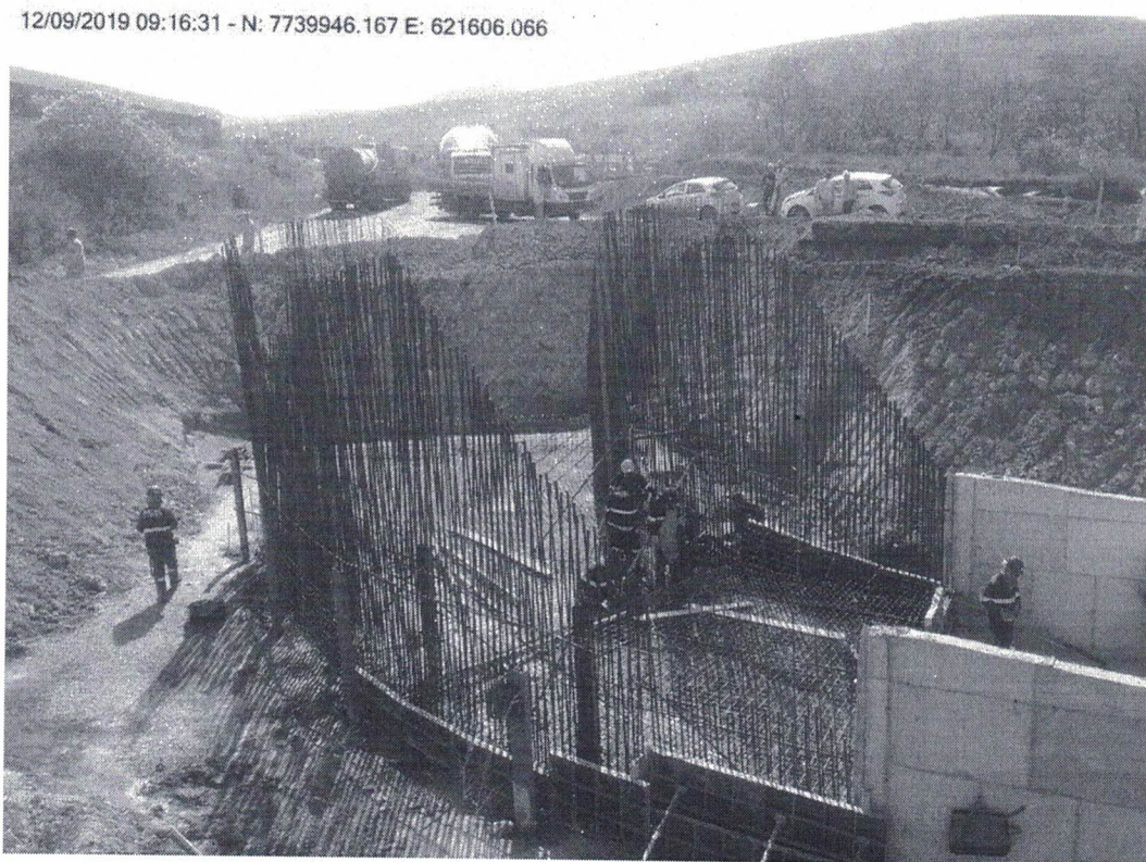
Foto 6- Execução da armação em trecho parcial do canal extravasor
