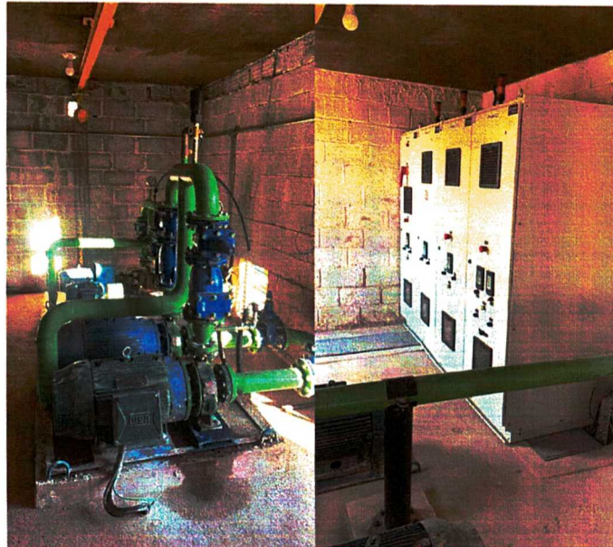
INVESTIMENTOS EM EQUIPAMENTOS HIDROMECÂNICOS – CAIXA 600 (DEPOIS)
