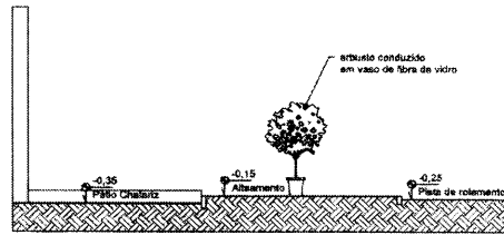
○ CORTE B-B esc 1/100
