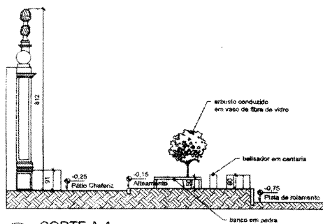
○ CORTE A-A esc 1/100
